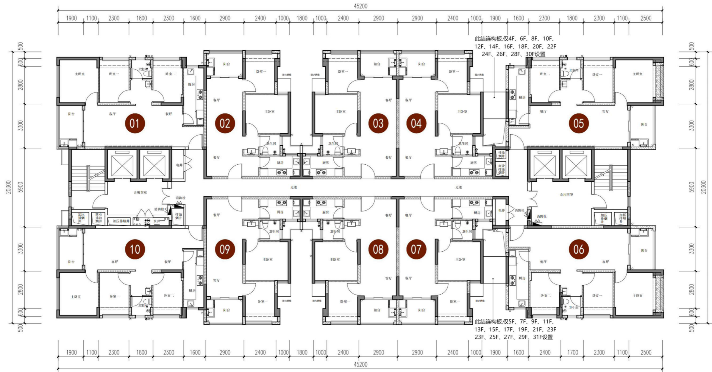
2 栋 4-31 层平面图
