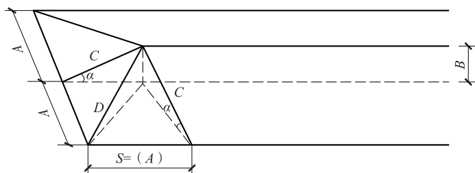
图 5.2.1 屋面坡度示意图
