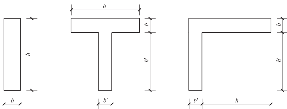
图 15.2.3 柱与墙划分方式示意图
