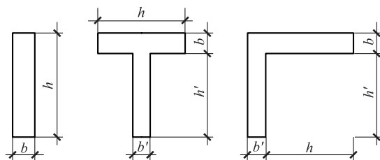
图 3.1.6 钢筋混凝土矩形柱、T 形柱、L 形柱尺寸标示图
