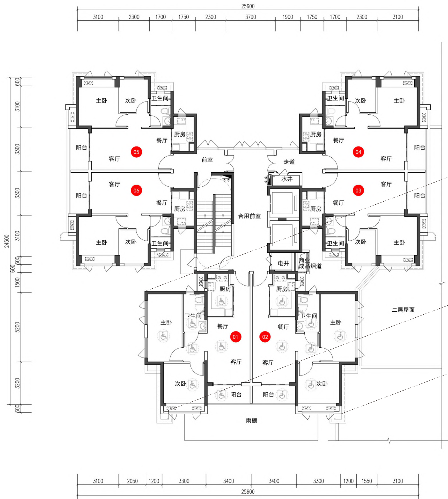
2栋一单元二层平面示意图
