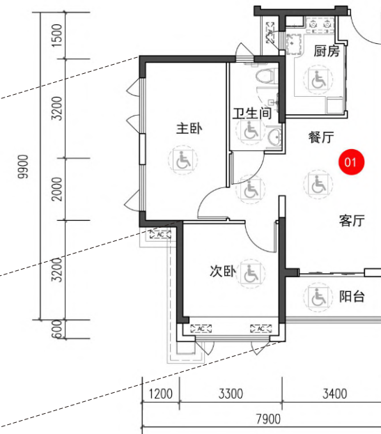
三层局部平面示意图
