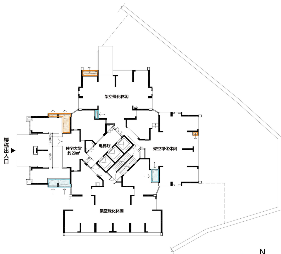
1栋安居型商品房首层平面图
