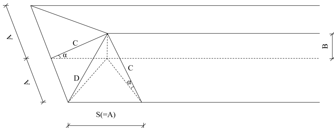
图 7.2.3 屋面坡度系数图
