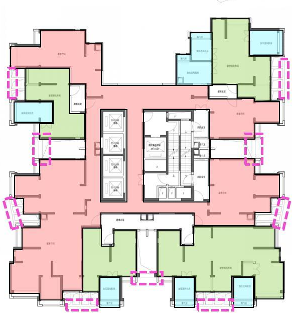
2栋一单元至六单元 避难层 (18F、35F)
