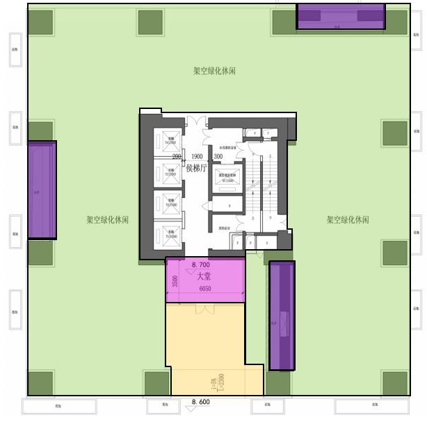
2栋四单元 架空层 (3F) 平面图
