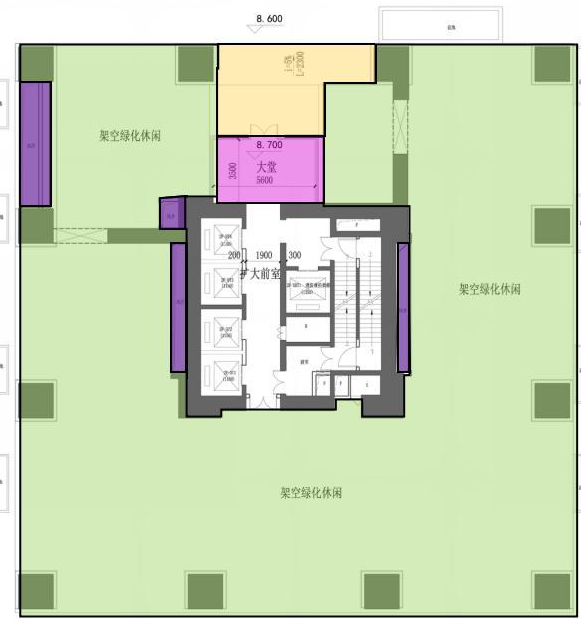
2栋六单元 架空层 (3F) 平面图
