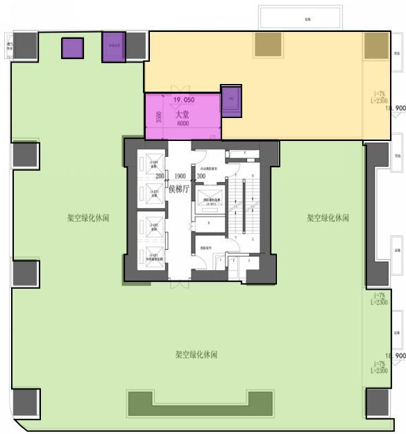
1栋一单元 架空层 (4F) 平面图
