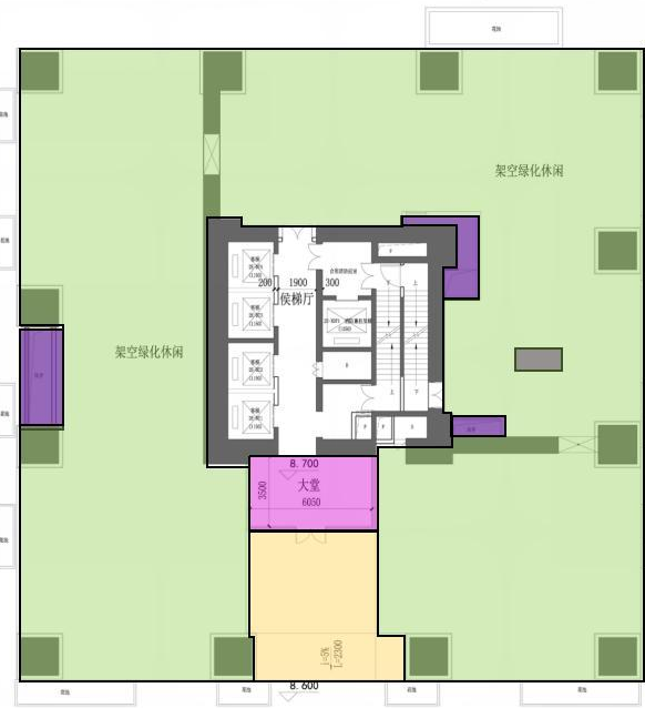
2栋五单元 架空层 (3F) 平面图
