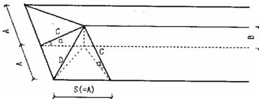
图4.2.1 屋面坡度示意图
