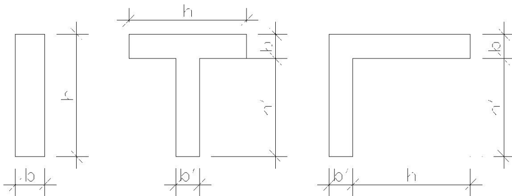
图7.2.3 柱与墙划分方式示意图
